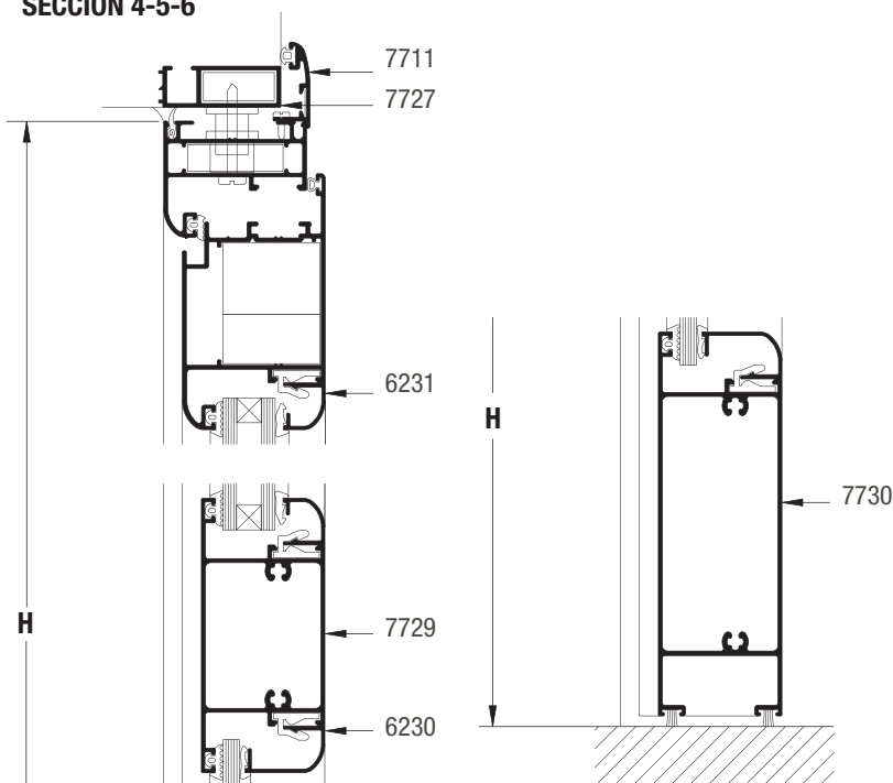
SECCION 4-5-6
