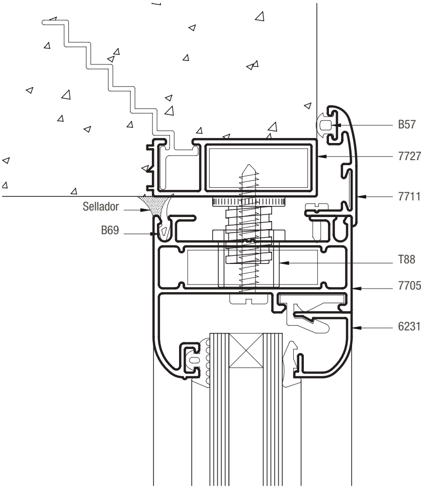
SECCION 3-4
