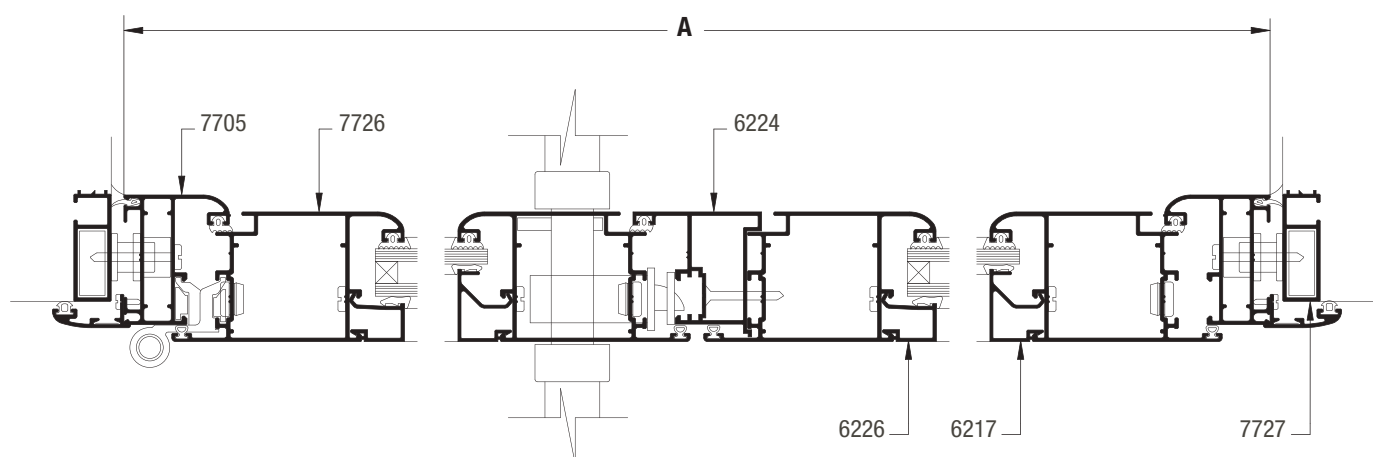
SECCION 1-2-3
