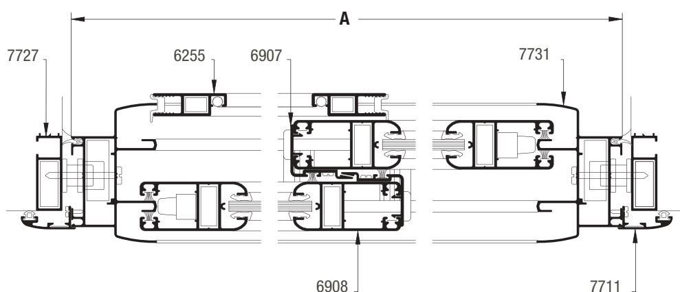
SECCION 1-2-3
